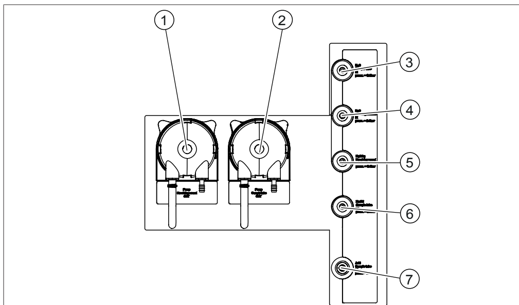
图 14: 后侧的接口
