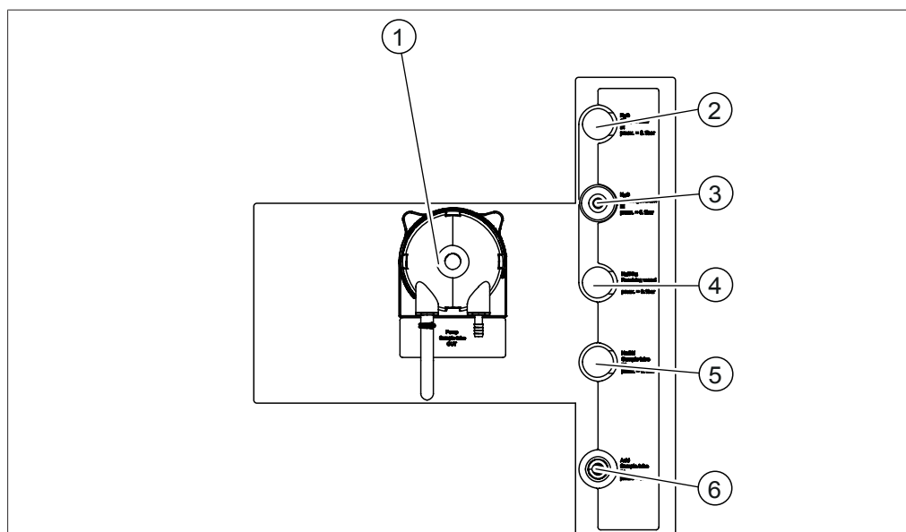
图 12: 后侧的接口
