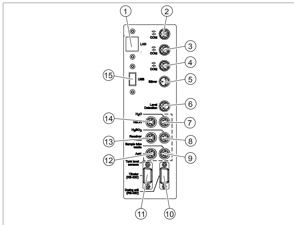
图 9: 通信连接
