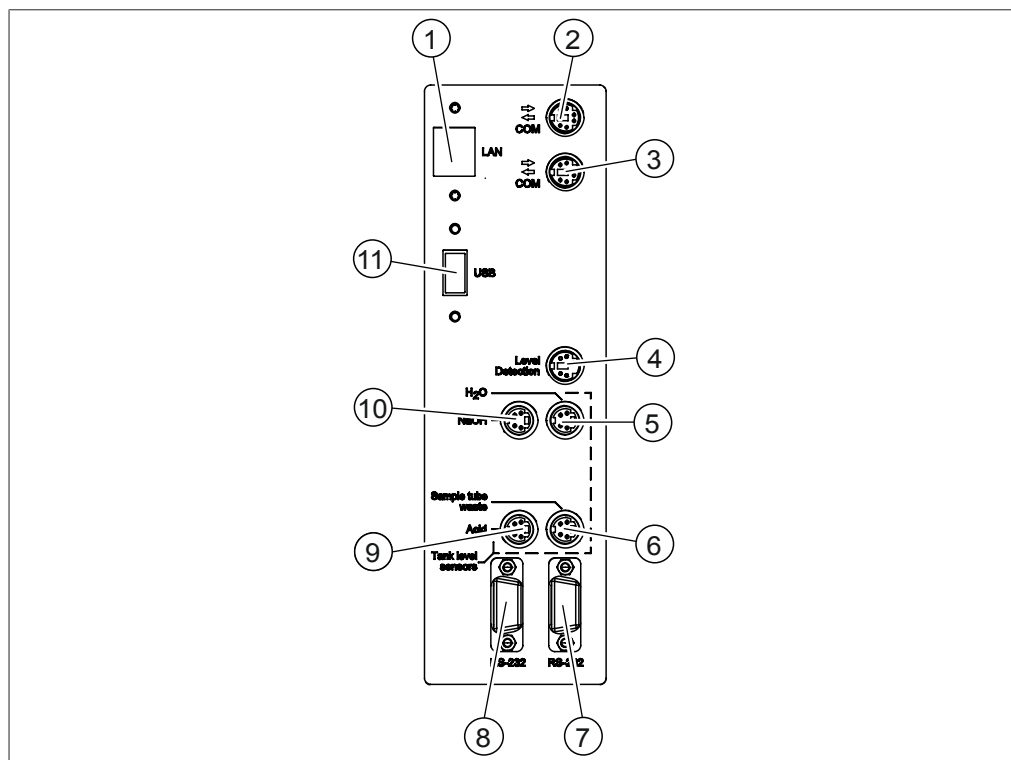
图 8: 通信连接
