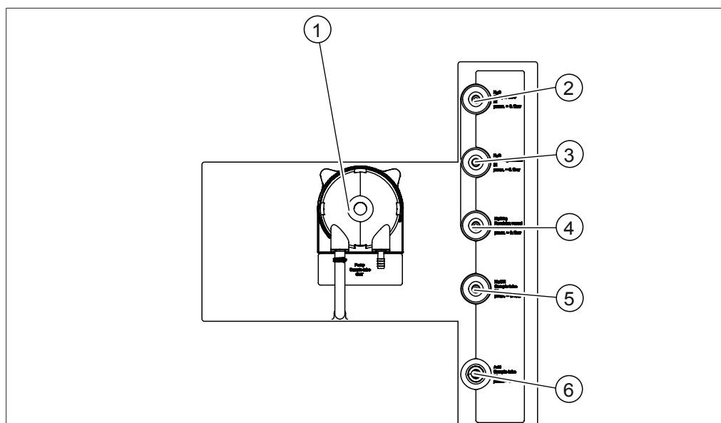
图 13: 后侧的接口
